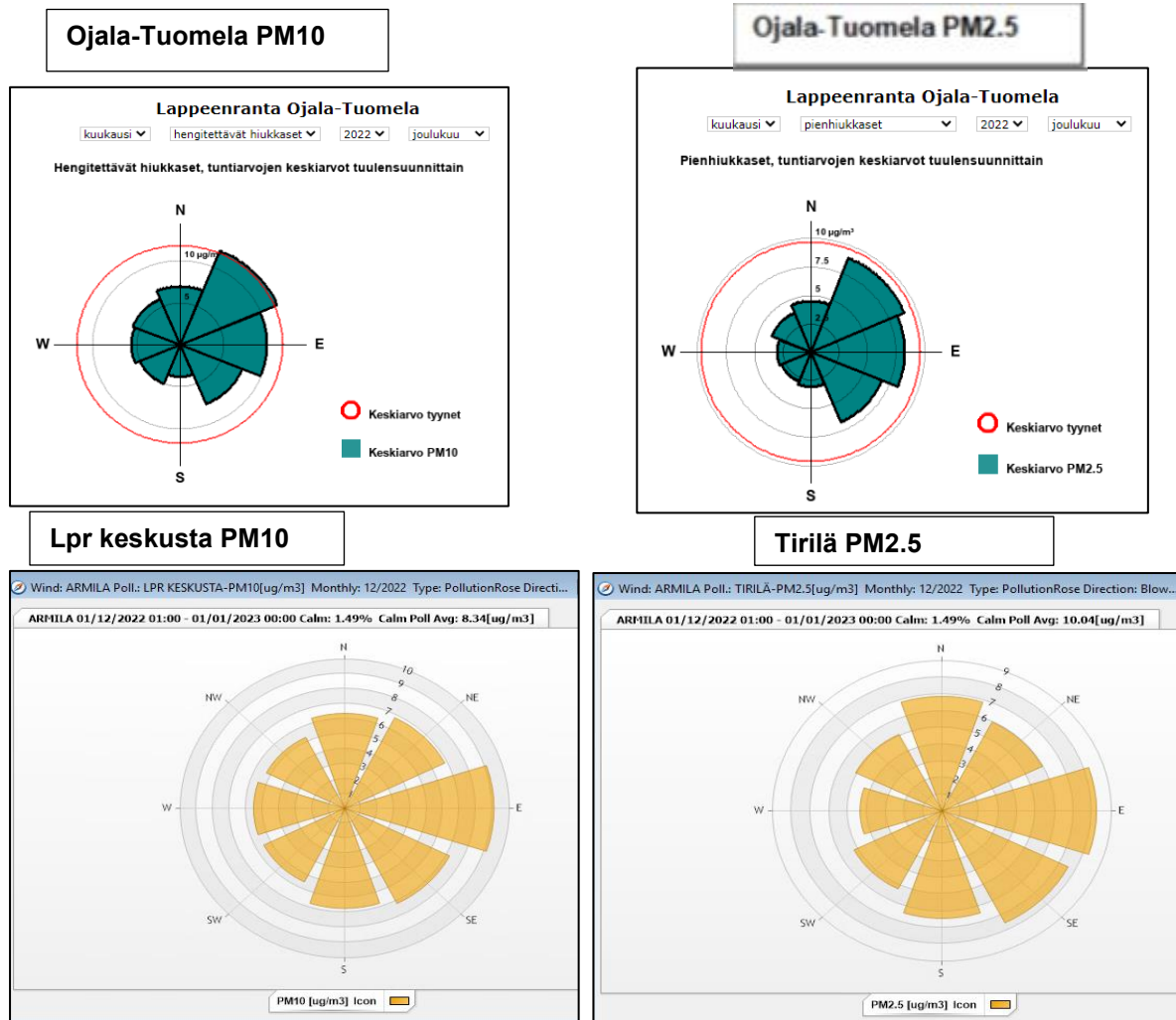
Kuva 11: IL:n ylläpitämän Ojala-Tuomela-mittauspisteen PM10- ja PM2.5- pitoisuusruusut, sekä Lappeenrannan keskustan kiinteän mittausaseman PM10-pitoisuusruusu ja Tirilän kiinteän mittausaseman PM2.5-pitoisuusruusu joulukuussa 2022
