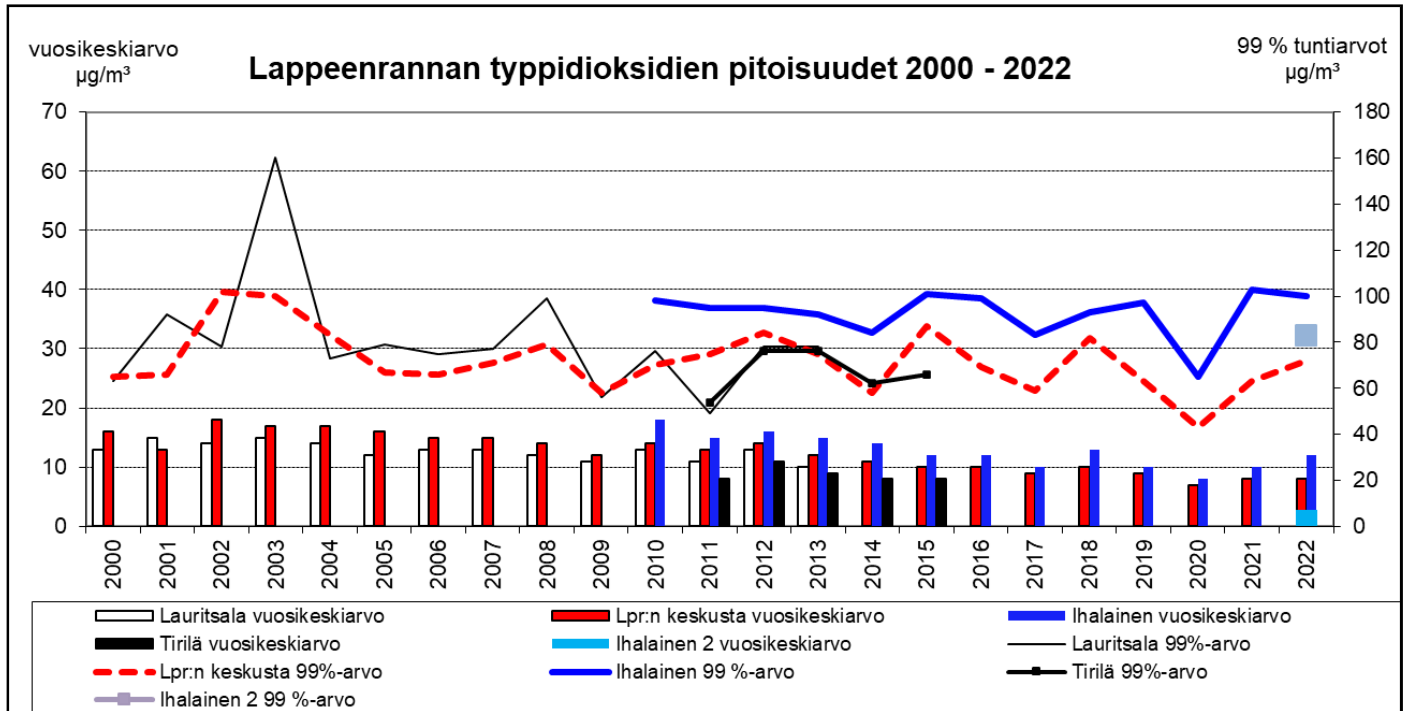
Kuva 49: Lappeenrannan mittauspisteiden NO 2 - vuosikeskiarvot ja 99 %:n suurimmat tuntiarvot vuosina 2000 - 2022 ( \mu\text{g}/\text{m}^3 ). Ihalaisessa mittauksia 1.1. – 30.5.2022 ja Ihalainen 2:ssa 7.7. – 31.12.2022
