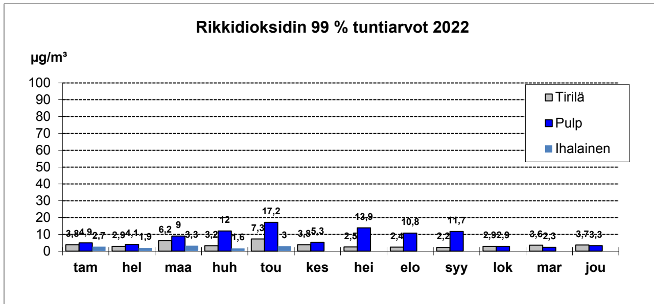
Kuva 12: Rikkidioksidin tuntiohjearvoon (250 µg/m 3 ) verrattavat pitoisuudet (99 % tuntikeskiarvot) vuoden 2022 aikana. Ihalaisen SO 2 -mittaus loppui 31.5.2022.
