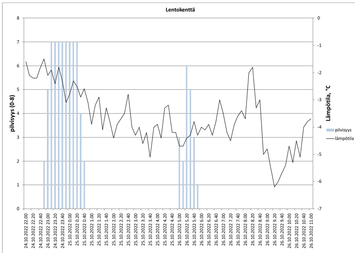
Kuva 3. Lämpötila ja pilvisuus
