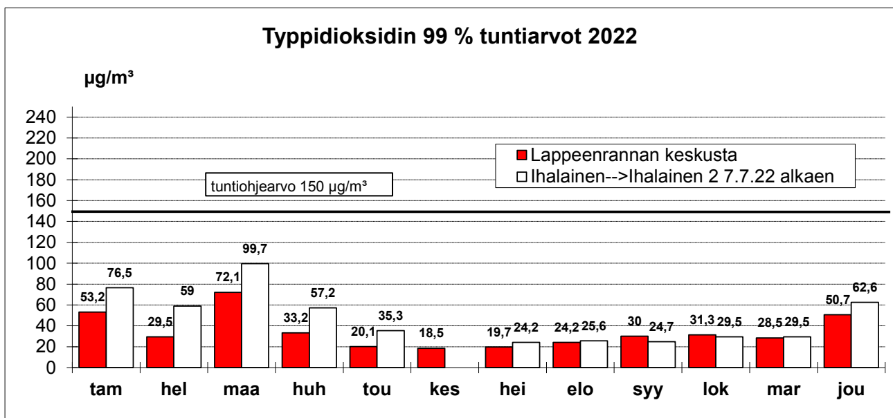
Kuva 14: Typpidioksidin tuntiohjearvoon (150 µg/m 3 ) verrattavat pitoisuudet (99 % tuntiarvot) vuonna 2022. Mittauspiste Ihalainen on nimetty Ihalainen 2:ksi 7.7.22 alkaen
