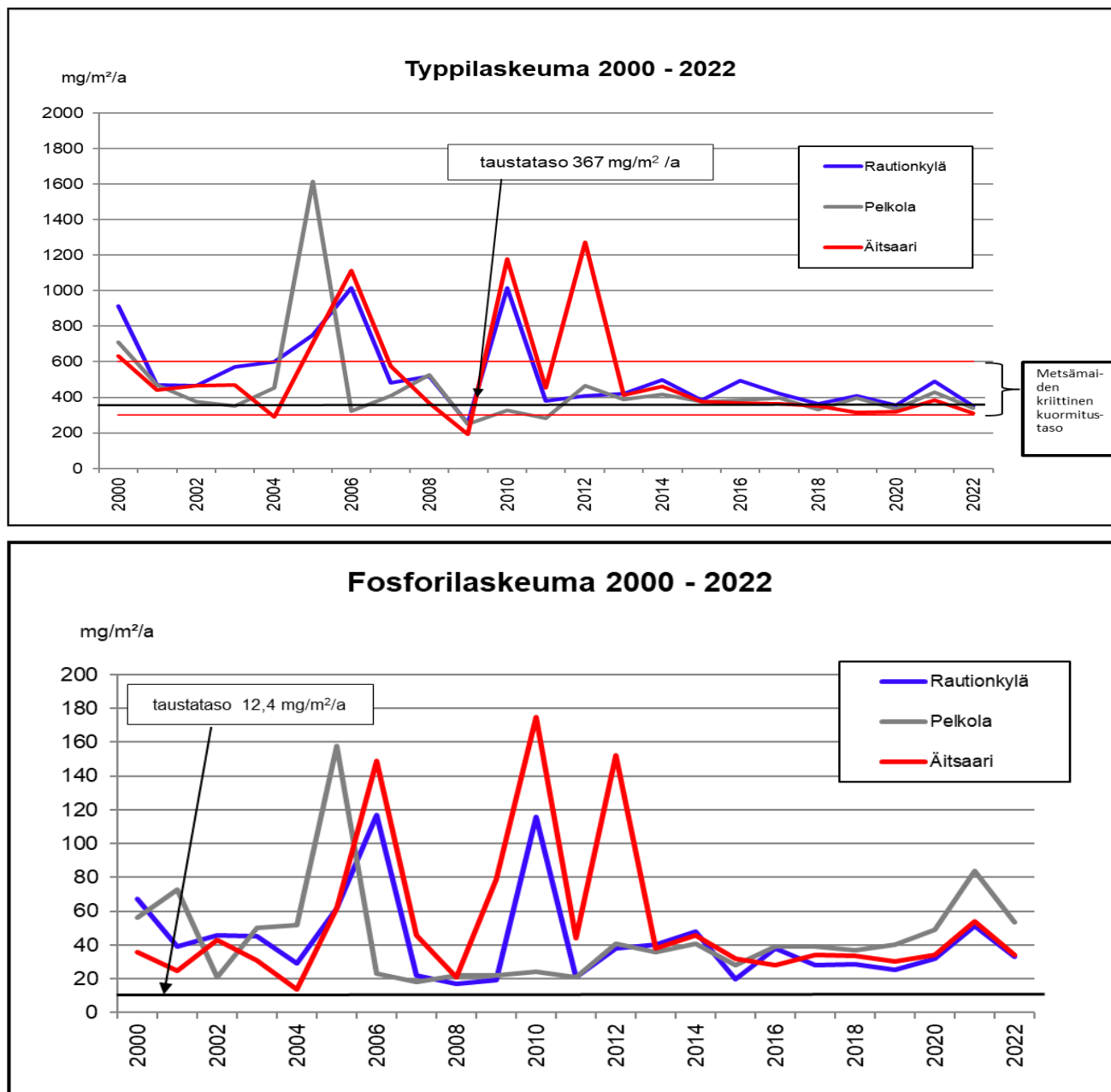
Kuva 33: Imatran laskeumapisteiden typpi- ja fosforilaskeumat vuosina 2000 - 2022
