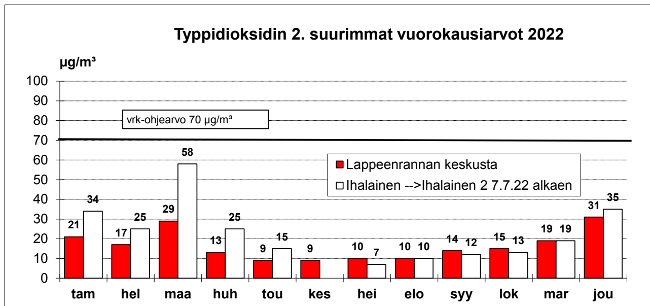
Kuva 13: Typpidioksidin vuorokausiohjearvoon (70 µg/m 3 ) verrattavat pitoisuudet (2. suurimmat vuorokausikeskiarvot) vuonna 2022. Mittauspiste Ihalainen on nimetty Ihalainen 2:ksi 7.7.22 alkaen
