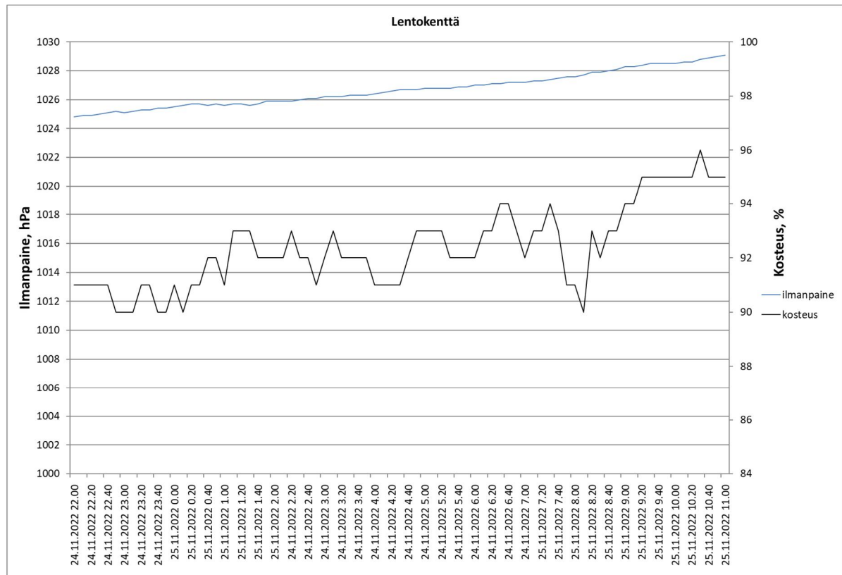
Kuva 2. Ilmanpaine ja kosteus
