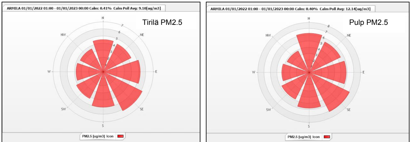
Kuva 58: Tirilän ja Pulpin PM2,5 - tuntikeskiarvojen tuulensuuntajakaumat sektoreittain vuonna 2022. Armilan tuulensuunta, tuulennopeus \geq 0,3 \text{ m/s} .
