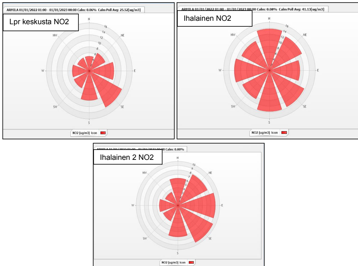
Kuva 47: Lappeenrannan keskustan, Ihalaisen ja Ihalainen 2:n NO 2 - tuntipitoisuuskaskeiavojen tuulensuuntajakauma sektoreittain vuonna 2022. Armilan tuulensuunta, tuulennopeus ≥ 0,3 m/s. Ihalaisessa mittauksia 1.1. – 30.5.2022 ja Ihalainen 2:ssa 7.7. – 31.12.2022
