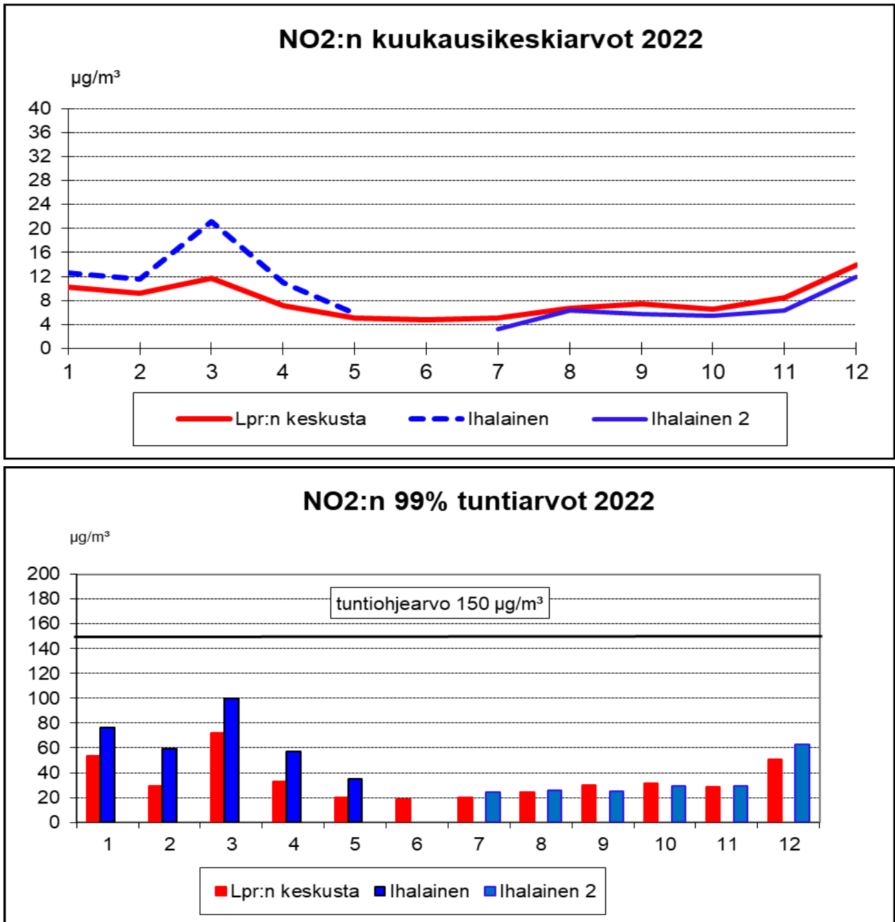
Kuva 48: Lappeenrannan mittauspisteiden NO 2 - kuukausikeskiarvot ja NO 2 - tuntiohjeeseen (99 % - tuntiarvot) verrattavat tunnusluvut vuonna 2022 (µg/m 3 ). Ihalaisessa mittauksia 1.1. – 30.5.2022 ja Ihalainen 2:ssa 7.7. – 31.12.2022
