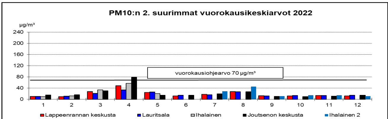
Kuva 50: Lappeenrannan keskustan, Lauritsalan, Ihalaisen ja Joutsenon keskustan PM10 - kuukausikeskiarvot ja kuukausien 2. suurimmat vuorokausikeskiarvot vuonna 2022 ( \mu\text{g}/\text{m}^3 ). Ihalaisessa mittauksia tammi-toukokuulta ja Ihalainen 2:ssa heinä-joulukuulta.
