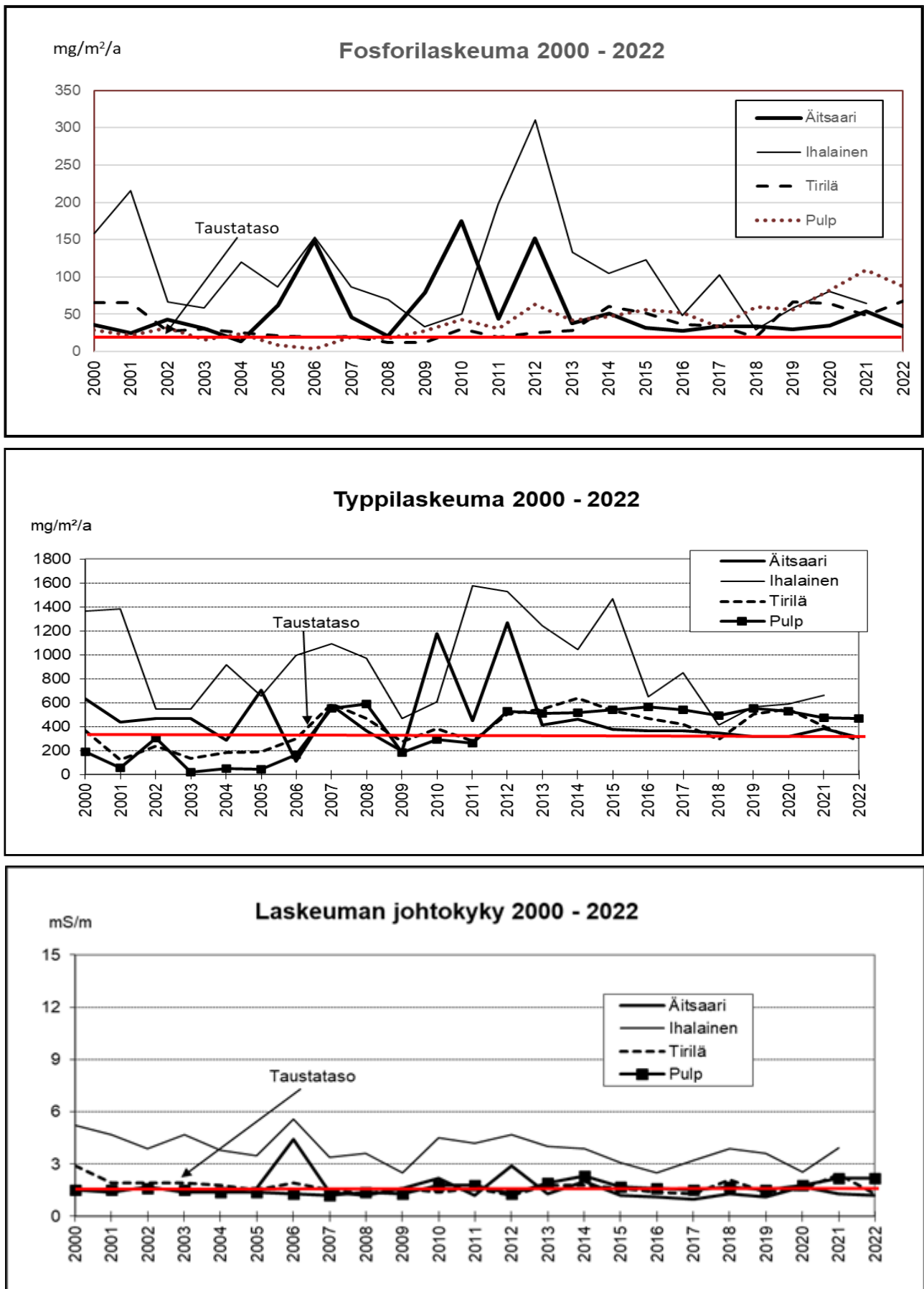
Kuva 61: Lappeenrannan mittauspisteiden laskeuman kokonaisfosforin, kokonaistypen ja johtokyvyn vuosilaskeumat 2000 – 2022. Ihalaisen arvo puuttuu, koska mittauspisteen paikkaa muutettiin kesäkuussa 2022.
