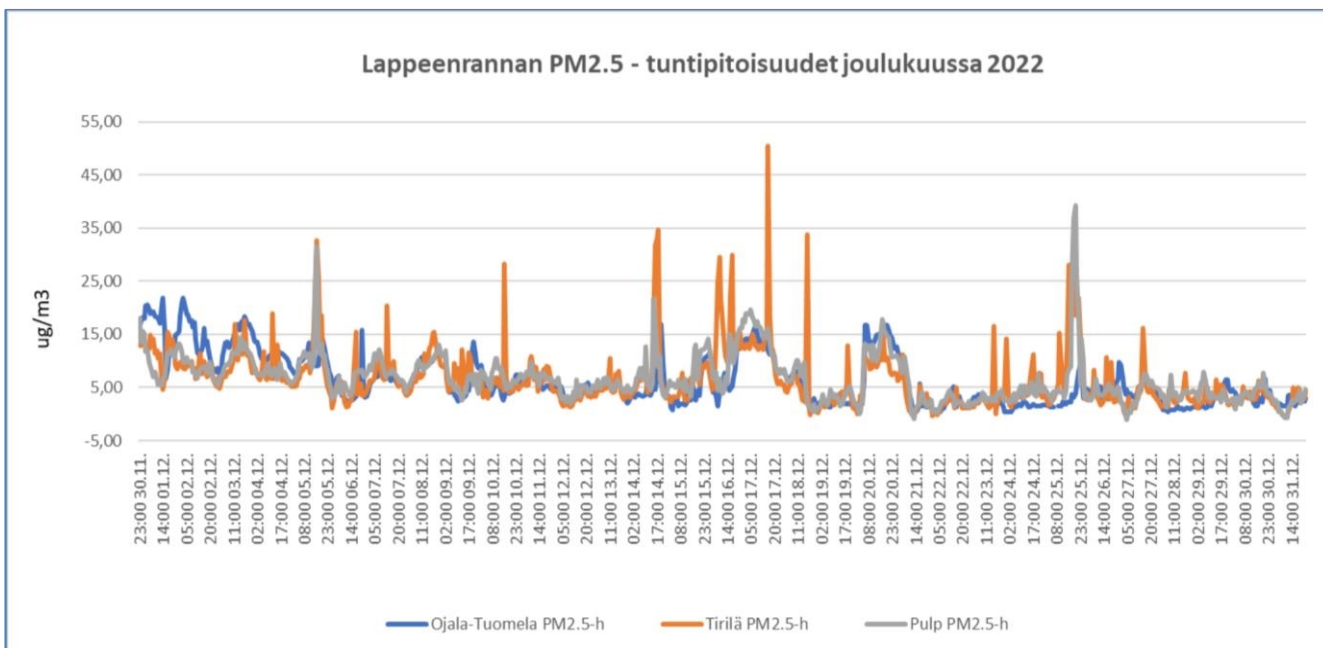
Kuva 9: IL:n ylläpitämän Ojala-Tuomela hiukkasmittauspisteen, ja Tirilän ja Pulpin kiinteiden mittauspisteiden PM2.5-tuntipitoisuudet joulukuussa 2022
