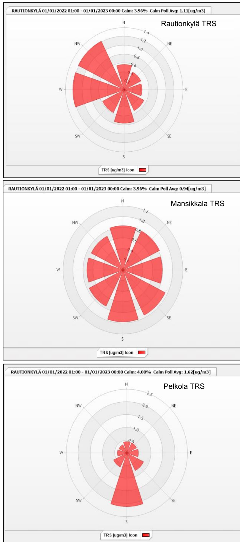
Kuva 12: Imatran Rautionkylän, Mansikkalan ja Pelkolan mittauspisteiden TRS-pitoisuuksien ( \mu\text{g}(\text{S})/\text{m}^3 ) tuulensuuntajakauma vuonna 2022. Rautionkylän sääaseman tuulensuunta, tuulennopeus \geq 0,3 \text{ m/s}
