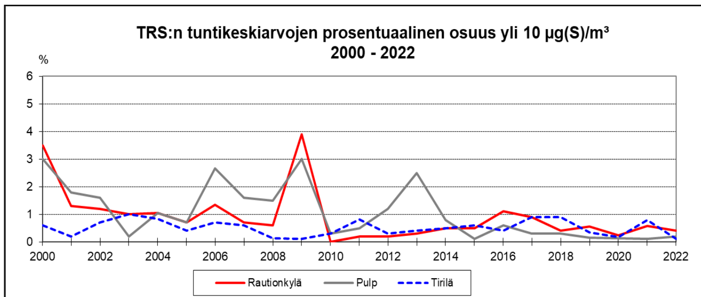
Kuva 64: TRS:n yli 10 \mu\text{g}(\text{S})/\text{m}^3 -tuntikeskiarvopitoisuuksien prosentiosuudet 2000 - 2022 Rautionkylässä, Pulpilla ja Tirilässä
