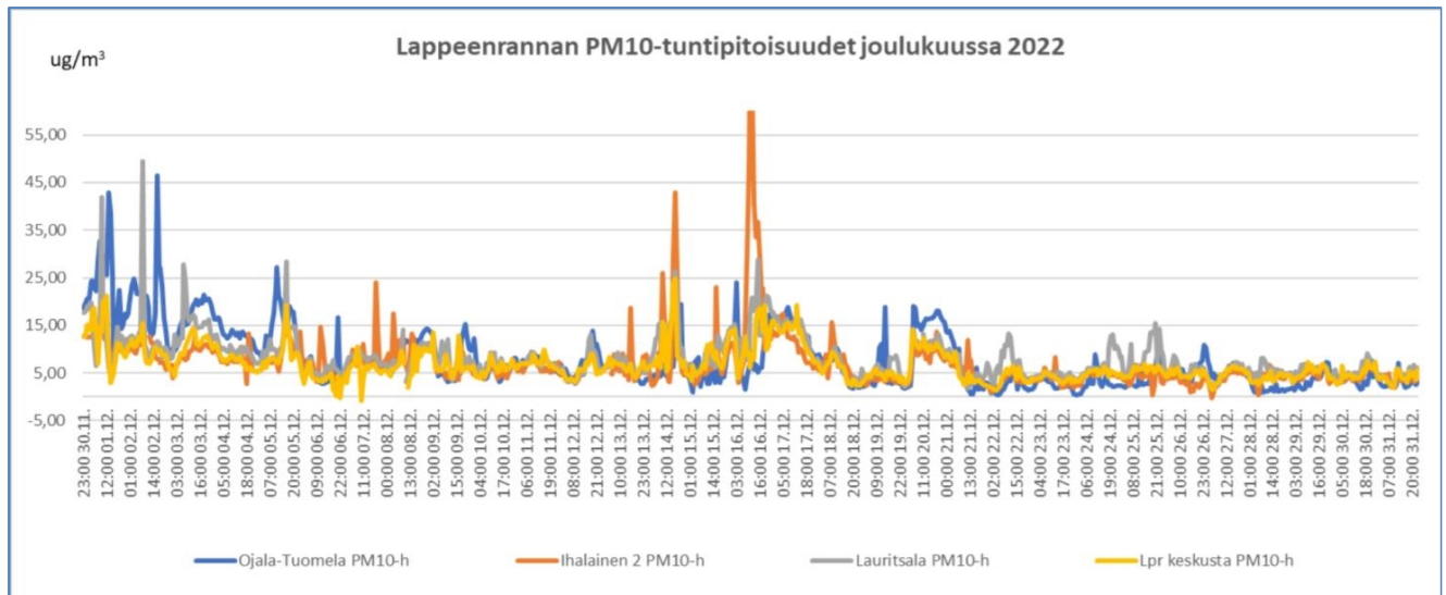
Kuva 5: IL:n ylläpitämän Ojala-Tuomelan hiukkasmittauspisteen sekä Ihalainen 2:n, Lauritsalan ja Lpr keskustan kiinteiden mittauspisteiden PM10-tuntipitoisuudet joulukuussa 2022.
