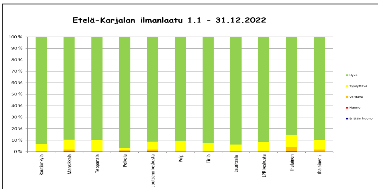
Kuva 62: Etelä-Karjalan ilmanlaatu eri mittauspisteillä tunti-indekseillä kuvattuna vuonna 2022. Ihalaisen indeksitiedot ovat 1.1. – 30.5.2022, ja Ihalainen 2:n tiedot 8.7. – 31.12.2022.
