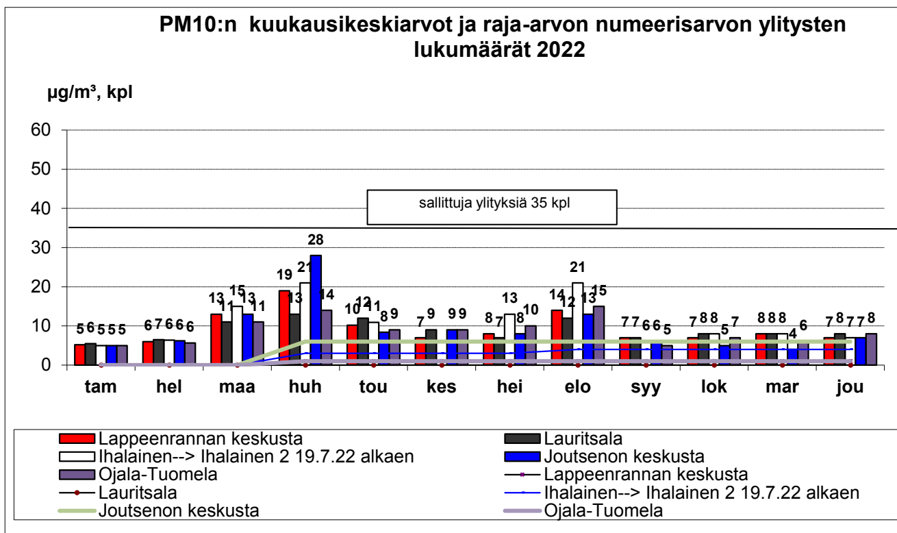
Kuva 8: PM10:en eli halkaisijaltaan alle 10 µm hiukkasten kuukausikeskiarvot (pylväsdiagrammi), sekä vuorokausiraja-arvon 50 µg/m³ ylitysten lukumäärä (sallittuja ylityksiä 35 kpl/vuosi) vuoden 2022 aikana (viivadiagrammi)
