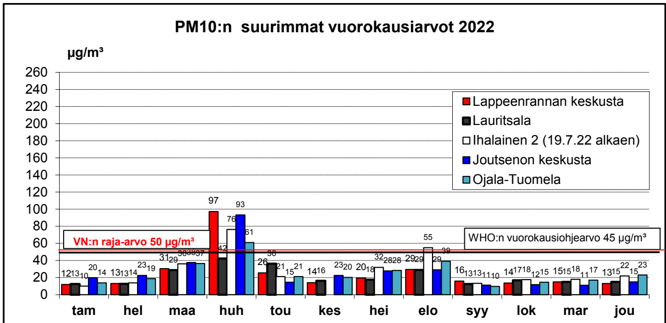
Kuva 7: PM10 – pitoisuuksien kuukausien suurimmat vuorokausikeskiarvot 2022 sekä WHO:n vuorokausiohjearvo 45 µg/ m 3 (sallittuja ylityksiä vuodessa 3) ja Suomen valtioneuvoston raja-arvo 50 µg/m 3 (sallittuja ylityksiä vuodessa 35). (Ihalainen → Ihalainen 2:n mittaukset alkoivat 19.7.22)
