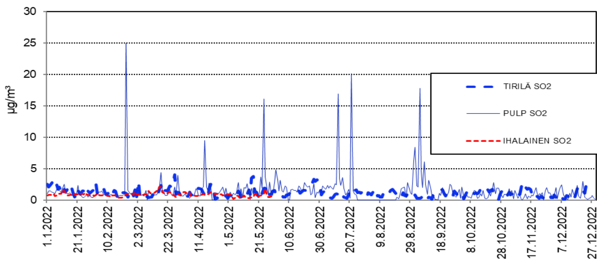
Kuva 43: Tirilän, Pulpin ja Ihalaisen mittauspisteiden rikkidioksidin vuorokausikeskiarvot vuonna 2022 ( \mu\text{g}/\text{m}^3 ). Ihalaisen rikkidioksidin mittaus loppui 30.5.2022.
