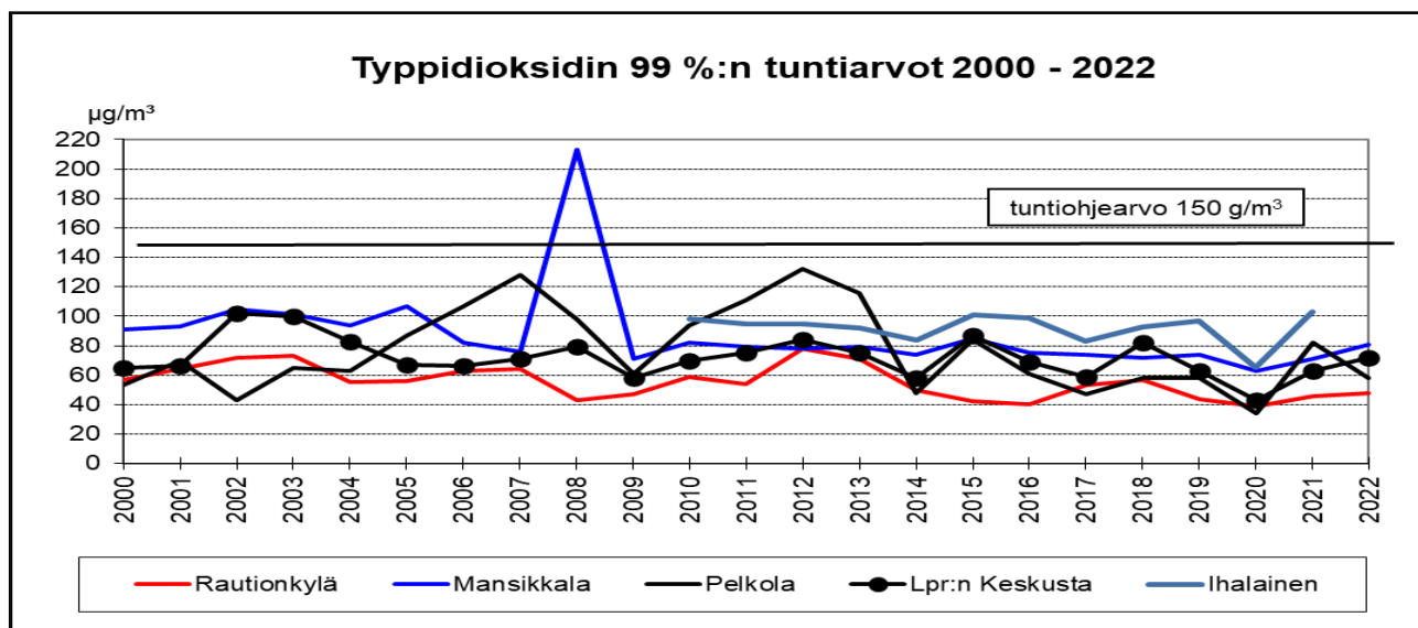
Kuva 71: Imatran ja Lappeenrannan mittauspisteiden typidioksidin tuntiojearvoon (150 µg/m³) verrattavat 99%-arvot vuosina 2000 – 2022 (µg/m³)
