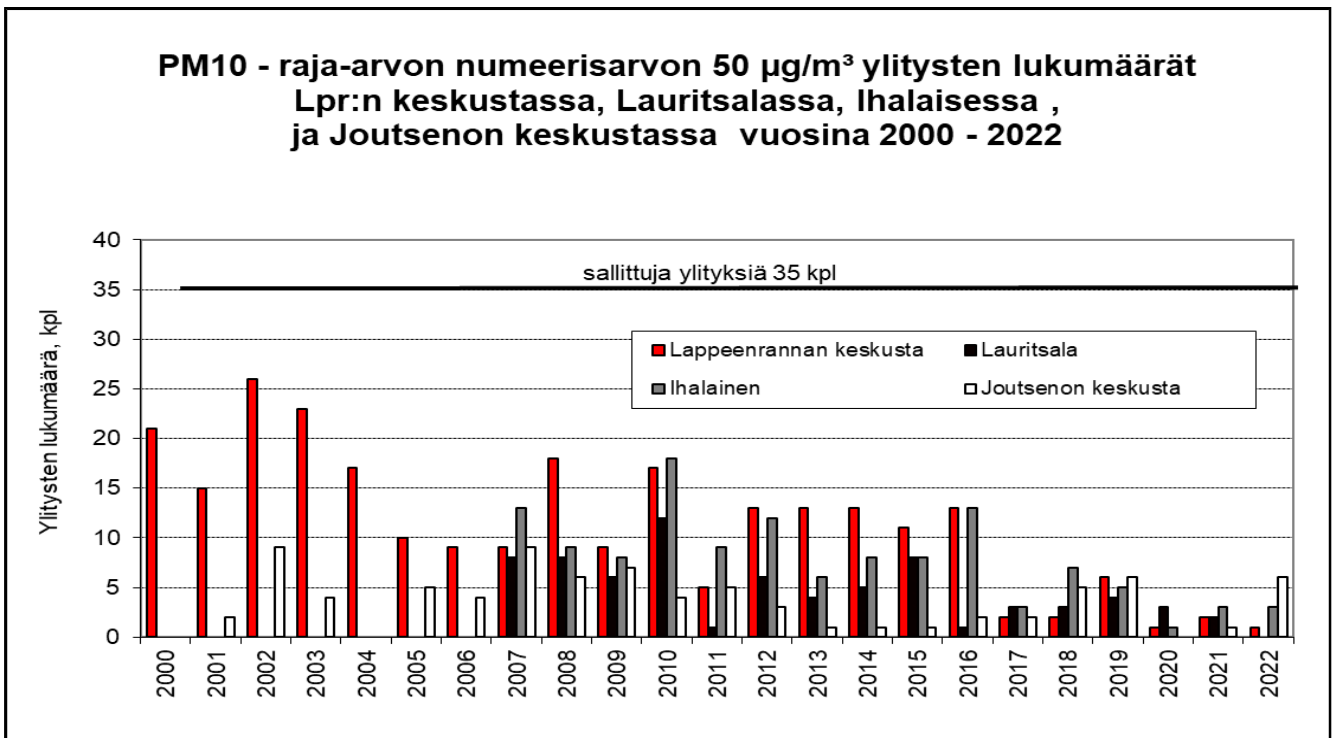
Kuva 52: Lappeenrannan hiukasmittauspisteiden PM10 - raja-arvon numeerisarvon 50 \mu\text{g}/\text{m}^3 ylitysten lukumäärät 2000 – 2022. Ihalaisessa mittauksia tammi-toukokuulta 2022.
