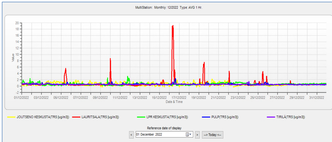
Kuva 2: Lappeenrannan mittauspisteiden TRS-tuntipitoisuudet joulukuussa 2022, \mu\text{g}(\text{S})/\text{m}^3
