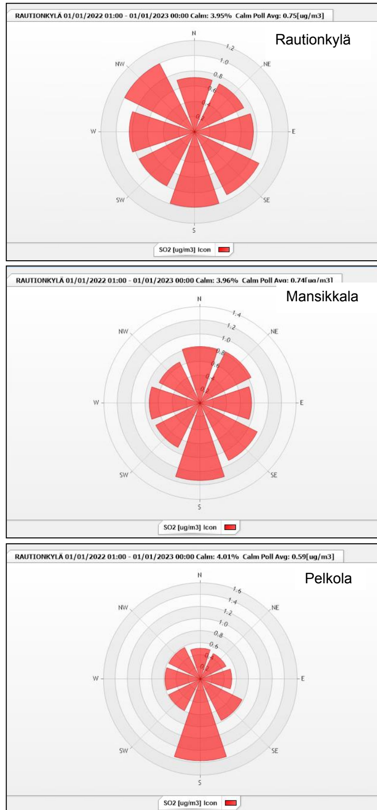
Kuva 17: Imatran Rautionkylän, Mansikkalan ja Pelkolan mittauspisteiden rikkidioksidipitoisuuksien ( \mu\text{g}/\text{m}^3 ) tuulensuuntajakaumat vuonna 2022. Rautionkylän tuulensuunta, tuulennopeus \geq 0,3 m/s.
