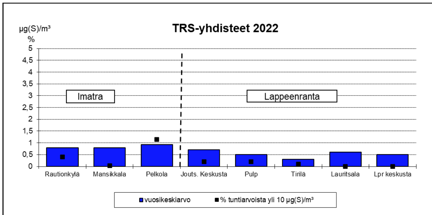
Kuva 63: Imatran ja Lappeenrannan mittauspisteiden vuoden 2022 TRS-yhdisteiden vuosikeskiarvot ja tuntipitoisuuden 10 \mu\text{g}(\text{S})/\text{m}^3 ylitysten %-osuudet
