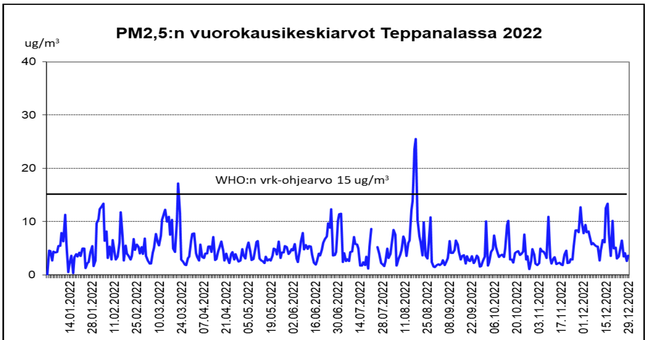
Kuva 26: Imatran Teppanalan PM2,5:n vuorokausikeskiarvot (µg/m³) vuonna 2022
