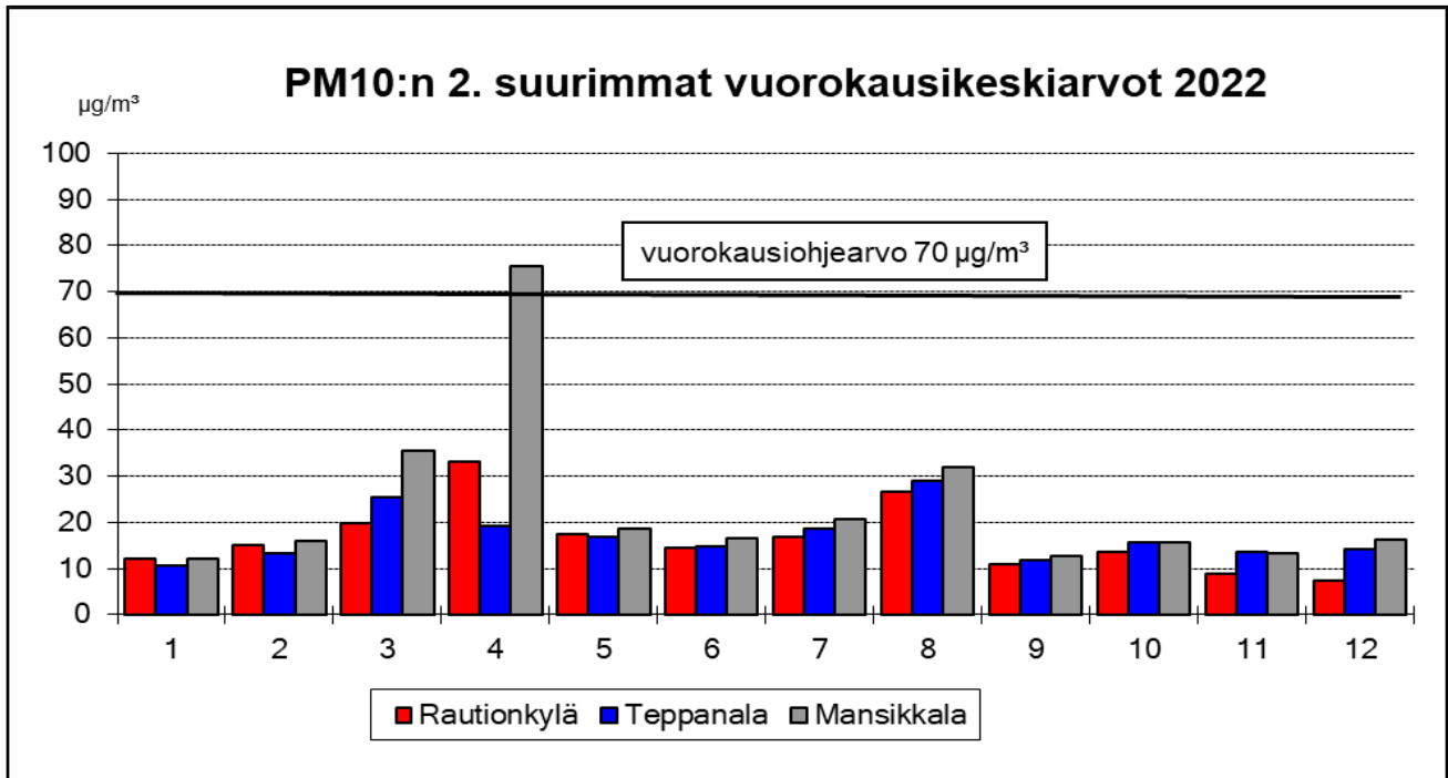
Kuva 25: Imatran mittauspisteiden PM10:n kuukausien 2. suurimmat vuorokausikeskiarvot (µg/m³) vuonna 2022
