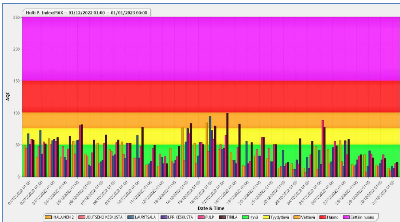
Kuva 1: Lappeenrannan ilmanlaadun mittausasemien vuorokausi-indeksit (vrk:n huonoin tunti-indeksi) joulukuussa 2022.
