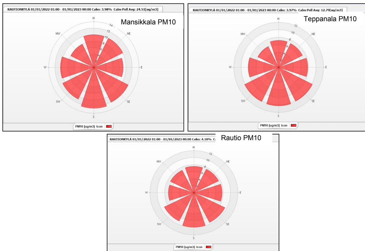
Kuva 27: Imatran Rautionkylän, Mansikkalan ja Teppanalan mittauspisteiden PM10:n pitoisuuksien tuulensuuntajakaumat vuonna 2022. Rautionkylän sääaseman tuulensuunta, tuulennopeus \geq 0,3 m/s.
