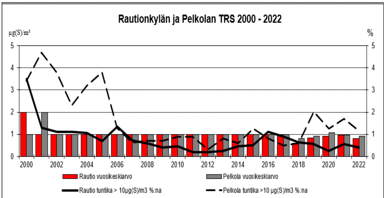
Kuva 14b: Rautionkylän ja Pelkolan TRS-yhdisteiden vuosikeskiarvot ja tuntikeskiarvon 10 µg(S)/m³ ylittäneiden tuntikeskiarvojen osuudet vuosina 2000–2022
