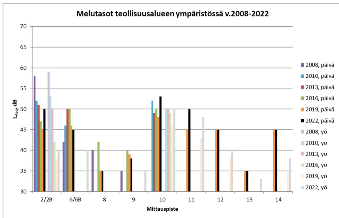
Kuva 4. Teollisuusalueen melutasot eri vuosina
