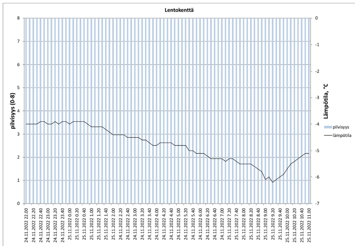
Kuva 3. Lämpötila ja pilvisuus
