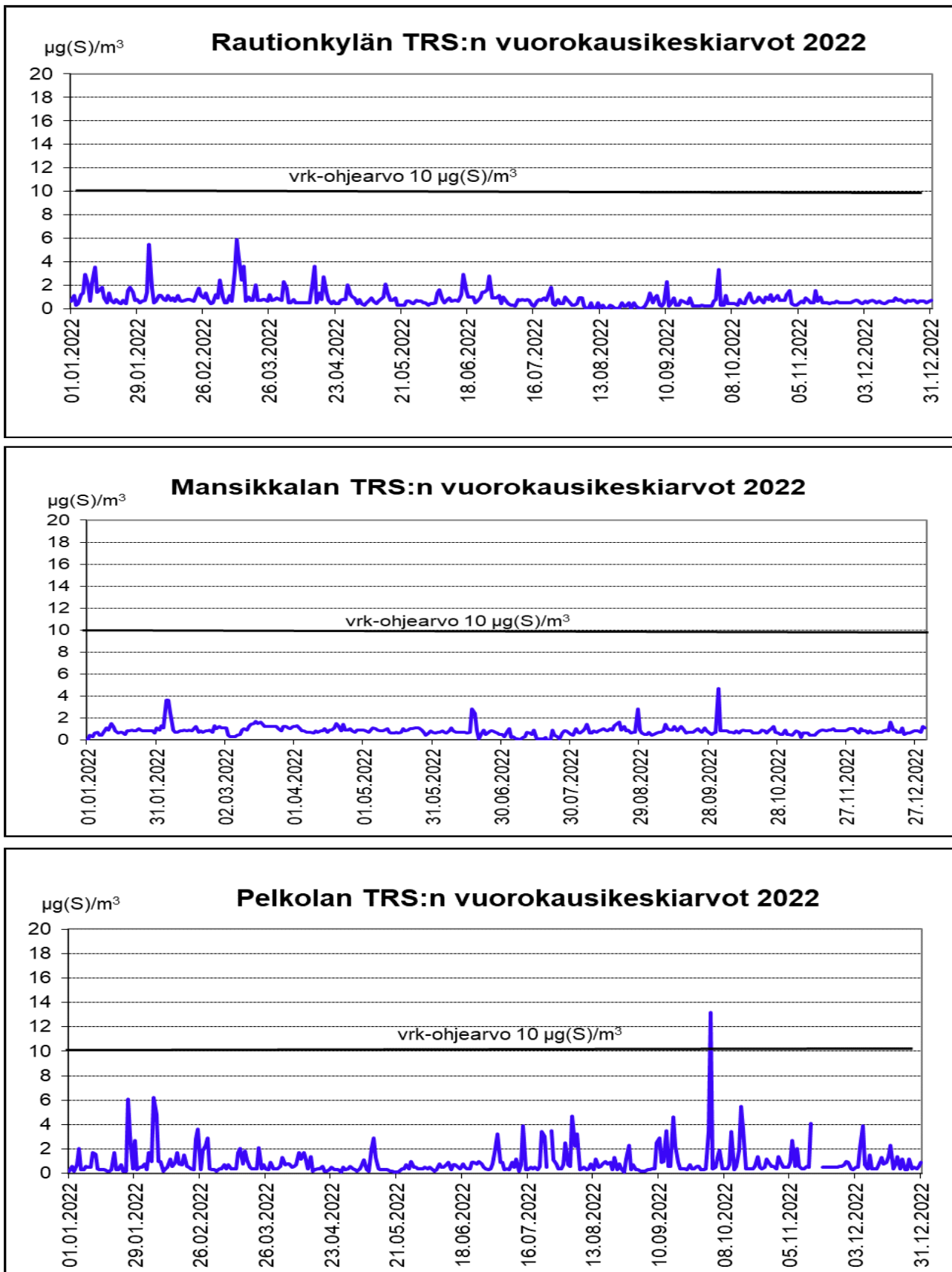
Kuva 11: Rautionkylän, Mansikkalan ja Pelkolan TRS-yhdisteiden vuorokausikeskiarvot ( \mu\text{g}(\text{S})/\text{m}^3 ) vuonna 2022
