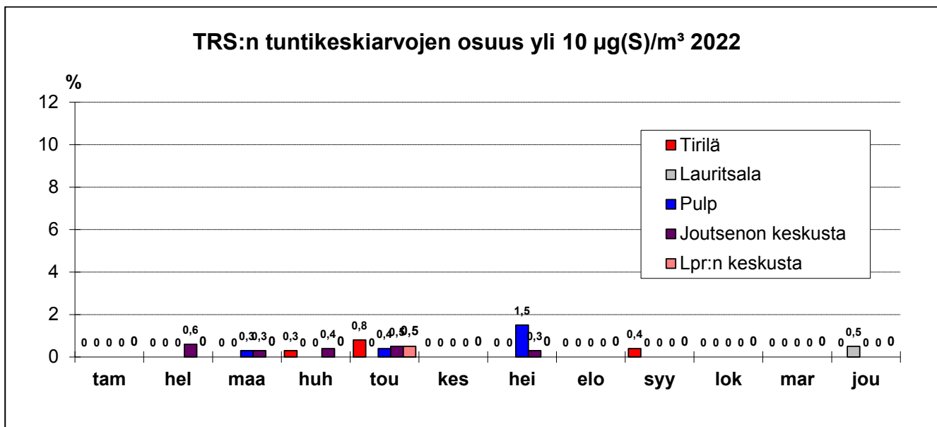
Kuva 4: TRS-yhdisteiden tuntikeskiarvon 10 µg(S)/m³ ylitysosuus (%) tuntikeskiarvoista vuonna 2022
