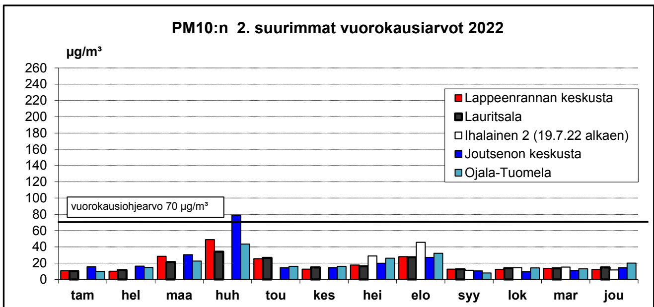
Kuva 6: PM10 - hiukkasten vuorokausiohjearvoon ( 70 \mu\text{g}/\text{m}^3 ) verrattavat pitoisuudet (kuukauden 2. suurimmat vuorokausikeskiarvot) 2022. Ihalainen 2:n mittaukset alkoivat 19.7.22.
