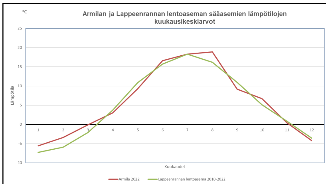
Kuva 9: Armilan sääaseman lämpötilojen kuukausikeskiarvot vuonna 2022 ja Lappeenrannan lentoaseman sääaseman lämpötilojen kuukausikeskiarvot vuosina 2010 – 2022
