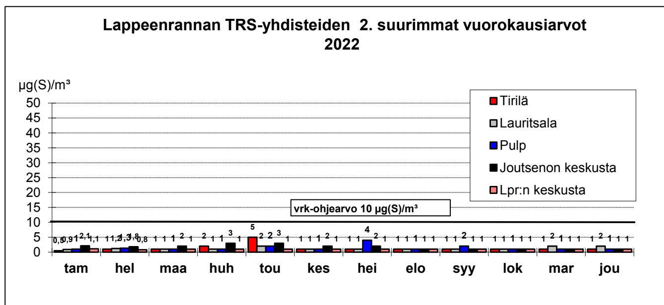
Kuva 3: TRS-yhdisteiden vuorokausiohjearvoon ( 10 \mu\text{g}(\text{S})/\text{m}^3 ) verrattavat pitoisuudet (2. suurimmat vuorokausikeskiarvot) vuonna 2022
