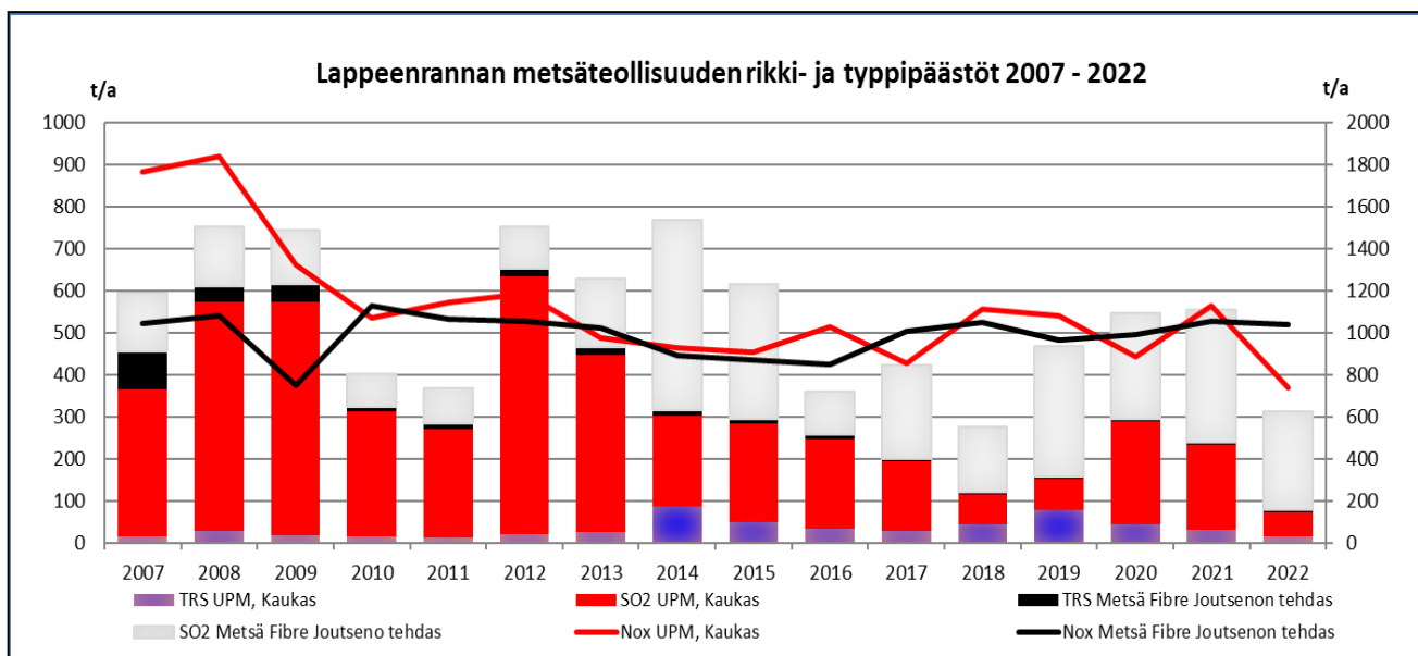
Kuva 4: Lappeenrannan tehtaiden TRS-, SO 2 - ja NO x - päästöt (t/a) vuosina 2007 - 2022 (Pylväsdiagrammien asteikko vasemmalla ja viivadiagrammien asteikko oikealla)
